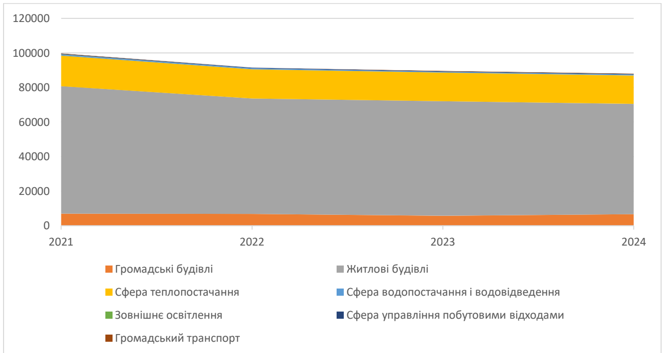
Рисунок 2.4.1. Зведений енергетичний баланс за категоріями кінцевих споживачів за 2021-2024 роки, МВт*год
