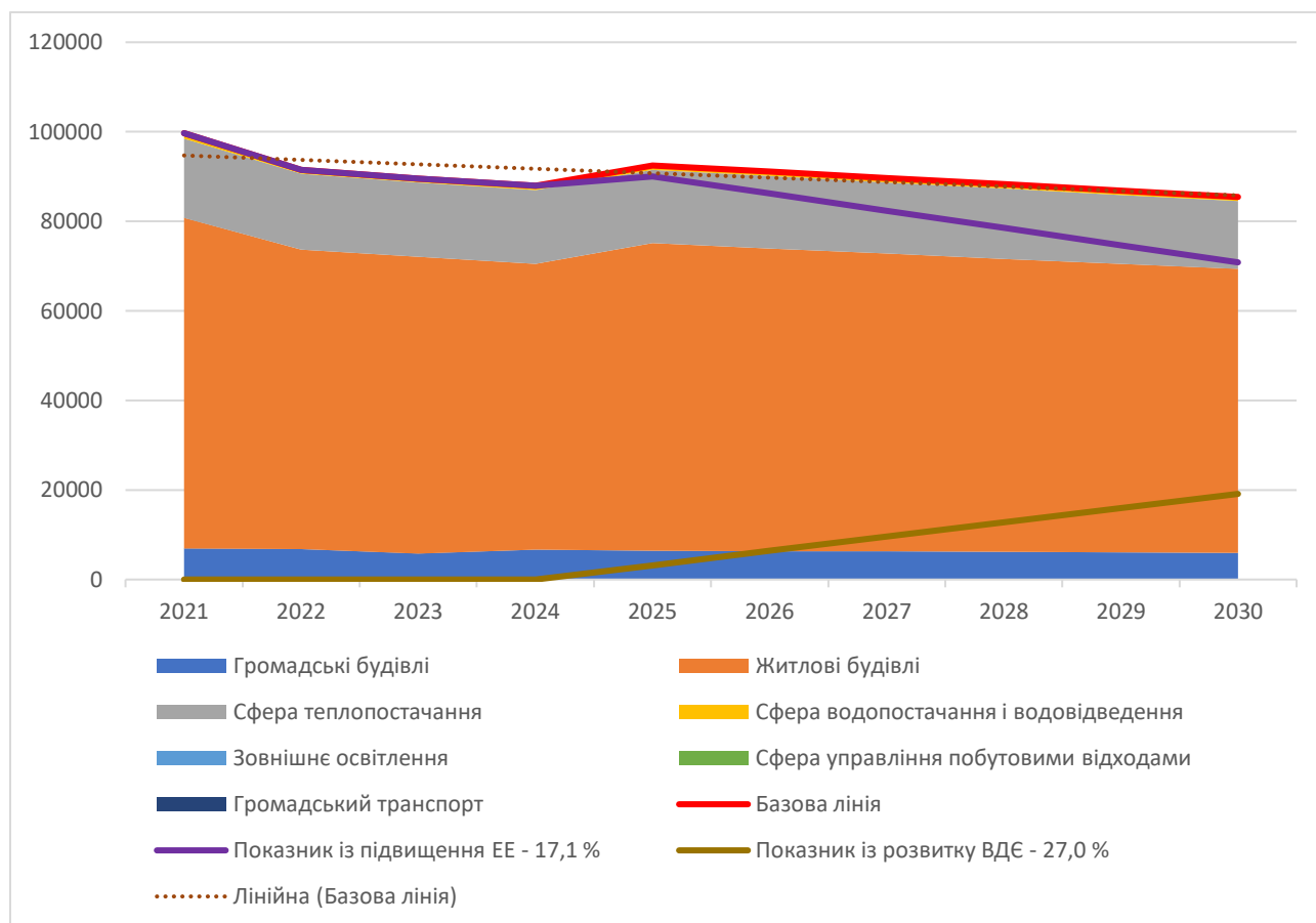
Рисунок 3.2.1. Базова лінія та цільові показники сталого енергетичного розвитку громади, МВт*год
